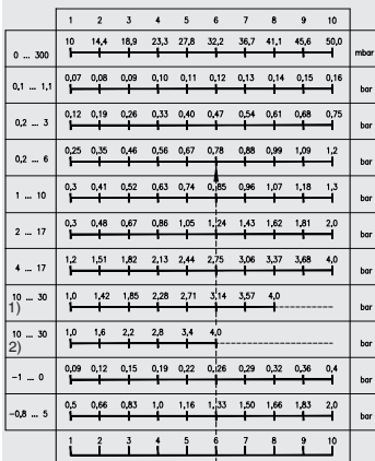
Nomogramă pentru număr setare
